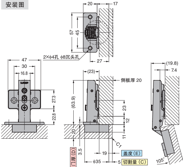
安装图
