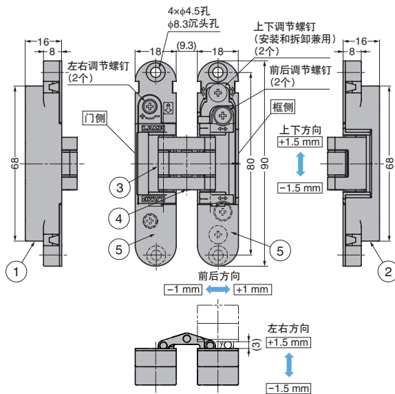
本图所示为拆下上侧螺钉盖后的状态。
